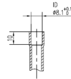
出气管详细 DISCHARGE TUBE
