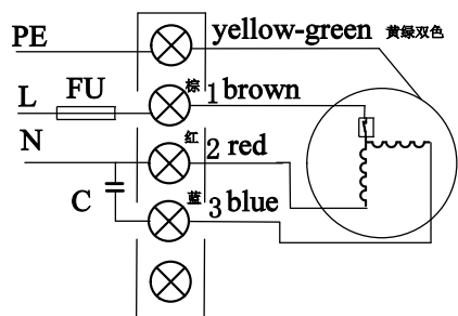
Wiring diagram:
